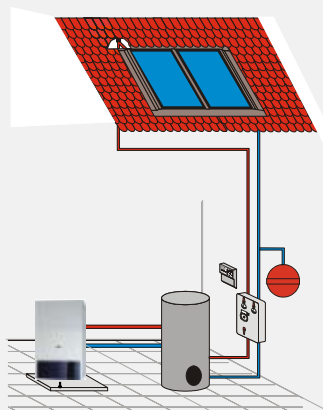
Schemat instalacji solarnej z kotłem kondensacyjnym
